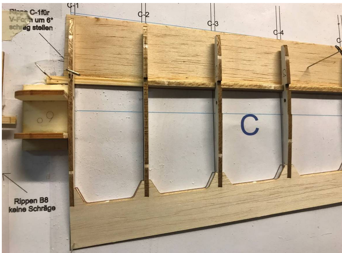
Rohbau Außenflügel, Schrägstellung der Rippe C1 beachten
