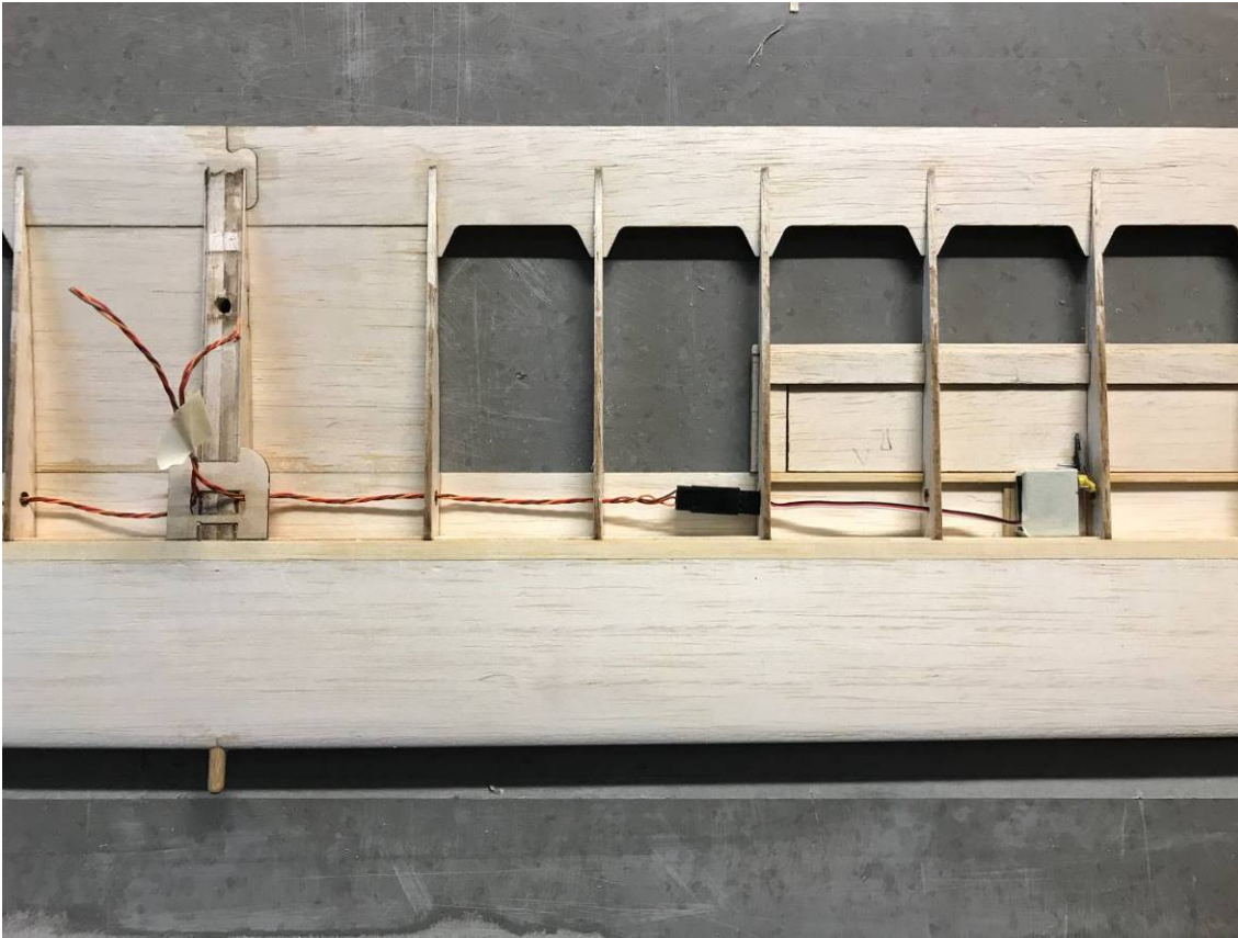
Kabelführung im Flügel
