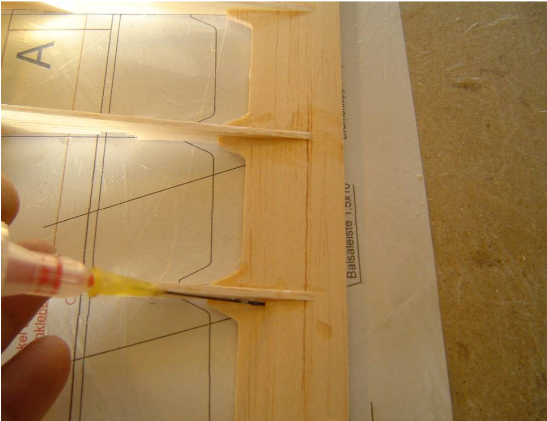
Verklebung der Endleiste
